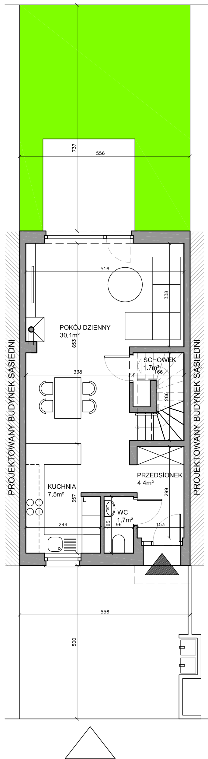
RZUT PARTERU
